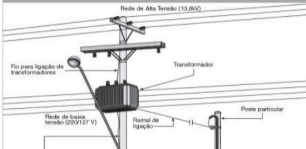
Figura 2.1 Fornecimento de energia elétrica (detalhes das ligações do ramal de entrada do consumidor).
